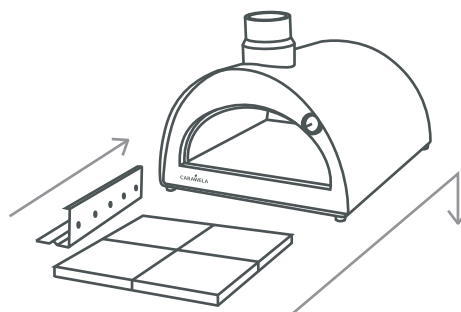
2 - Die feuerfesten Ziegeln und das Brennholzgestell einlegen
