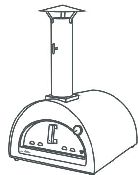
3 - Das Rauchrohr in die obere Öffnung einschieben und festschrauben
