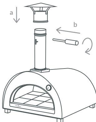
1 - Das Thermometer anschließen
